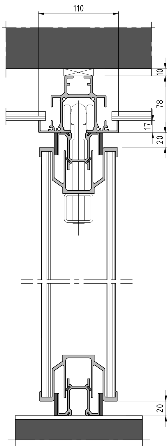
1-punts ophanging
